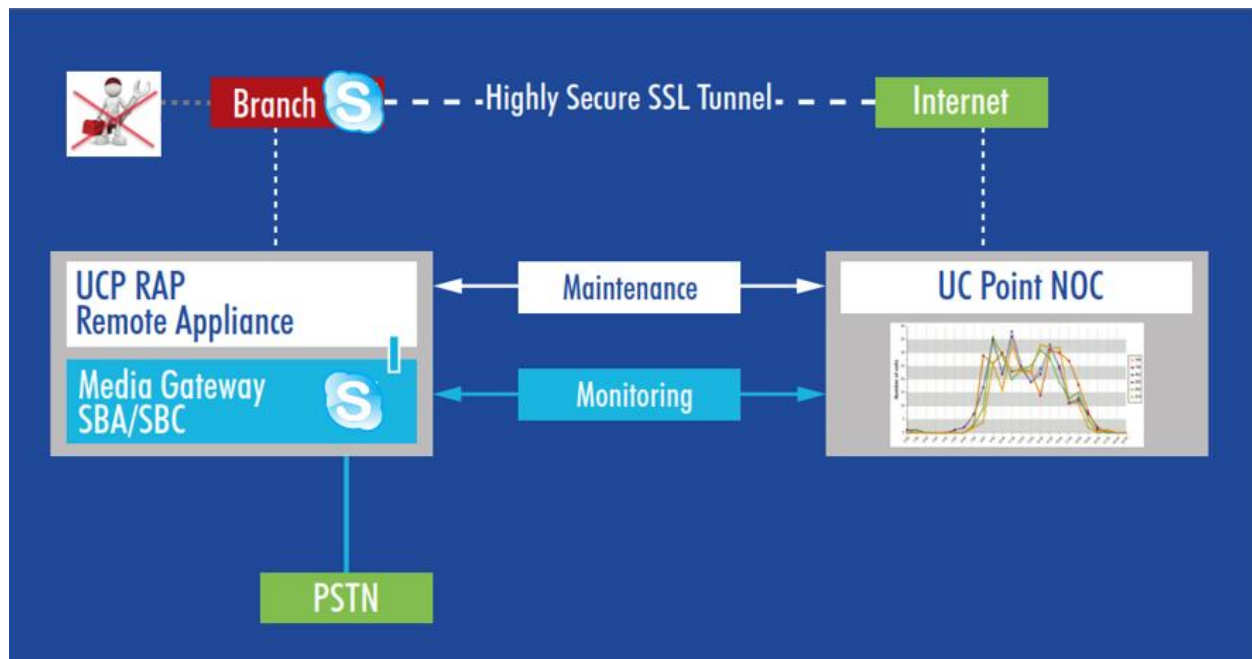
Grafik: Fernüberwachung einer UC-Infrastruktur
