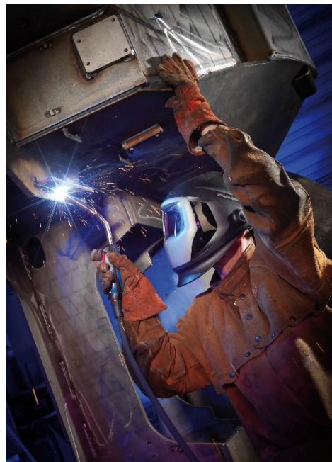
Der wassergekühlte MB EVO PRO 36 von ABICOR BINZEL in Aktion
