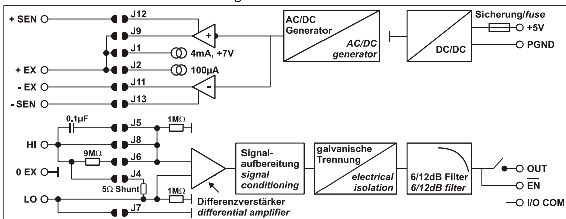
Funktionsschaltbild
