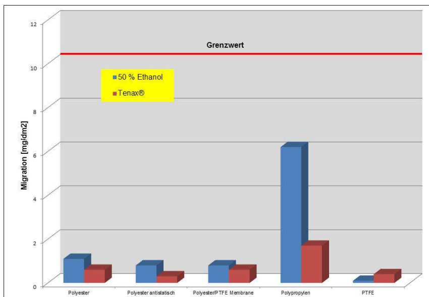
Abb. 3: Vergleich der Messwerte mit dem EU Grenzwert von 10 mg/dm 2
