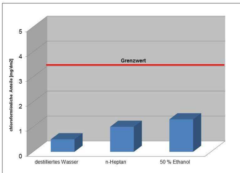
Abb. 4: Messergebnisse für Polyester gem. FDA Prüfvorschrift, Grenzwert 3,1 mg/dm 2
