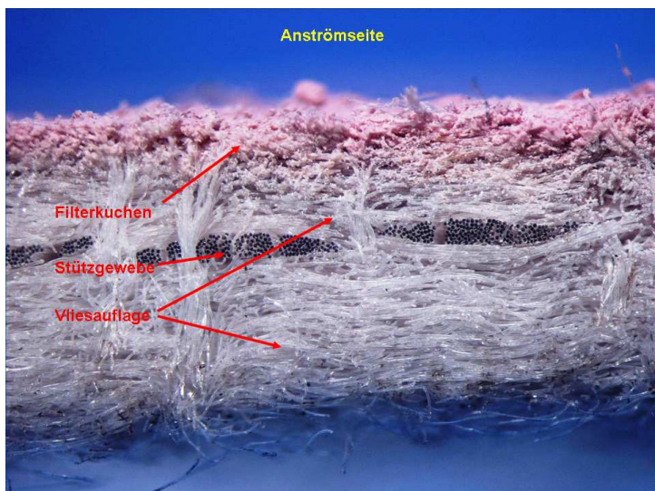
Abb. 1: Querschnitt eines gebrauchten Filtermediums mit an der Oberfläche angelagertem Filterkuchen
