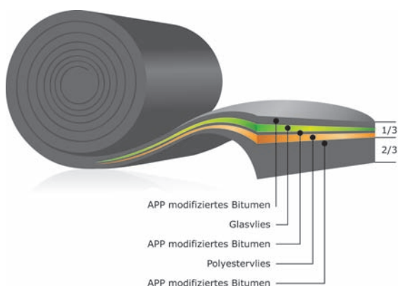
Bild 3: Aufbau der AirTex® F-TR
